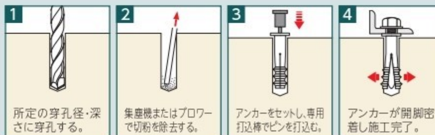
施工方法
